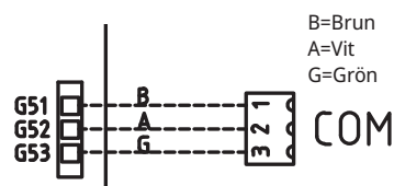
Detaljbild från elschema.
