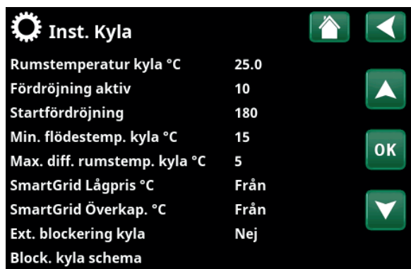
Meny "Avancerat/Inställningar/Kyla".
