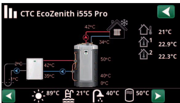
Huvudmenysidan för "Driftinfo" med vätska/vatten värmepump CTC EcoPart ansluten.
