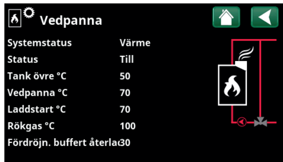
Meny "Driftinfo/Vedpanna".
