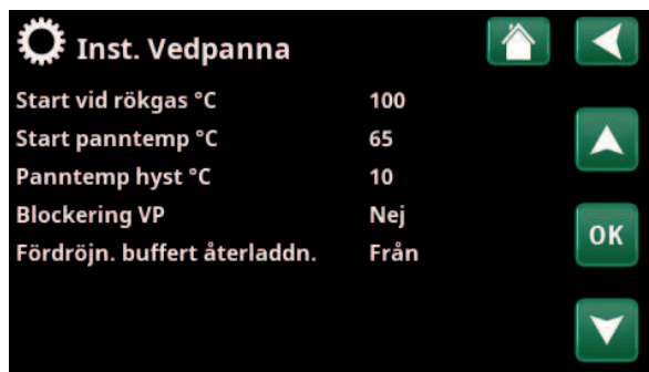
Meny "Avancerat/Inställningar/Vedpanna.
