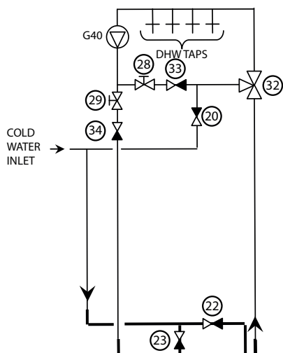
Bild 1. Varmvattencirkulation
