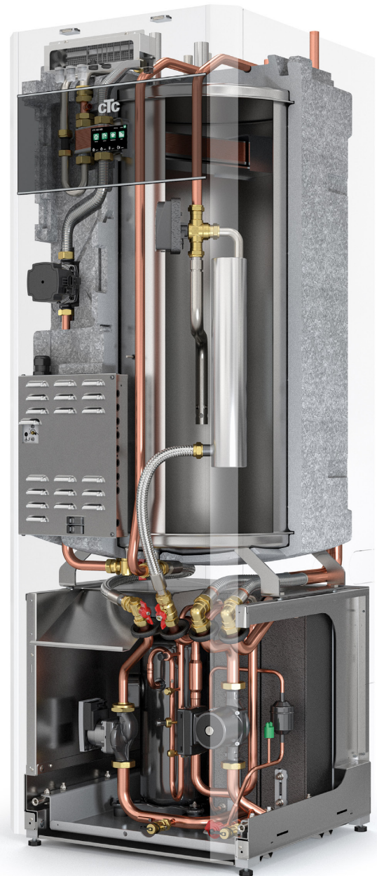
CTC GSi 600 Varvtalsstyrda värmepumpar för berg-, jord- eller sjövärme.
